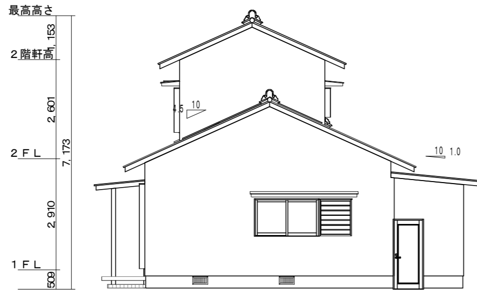
東側立面図
