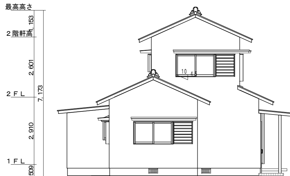
西側立面図
